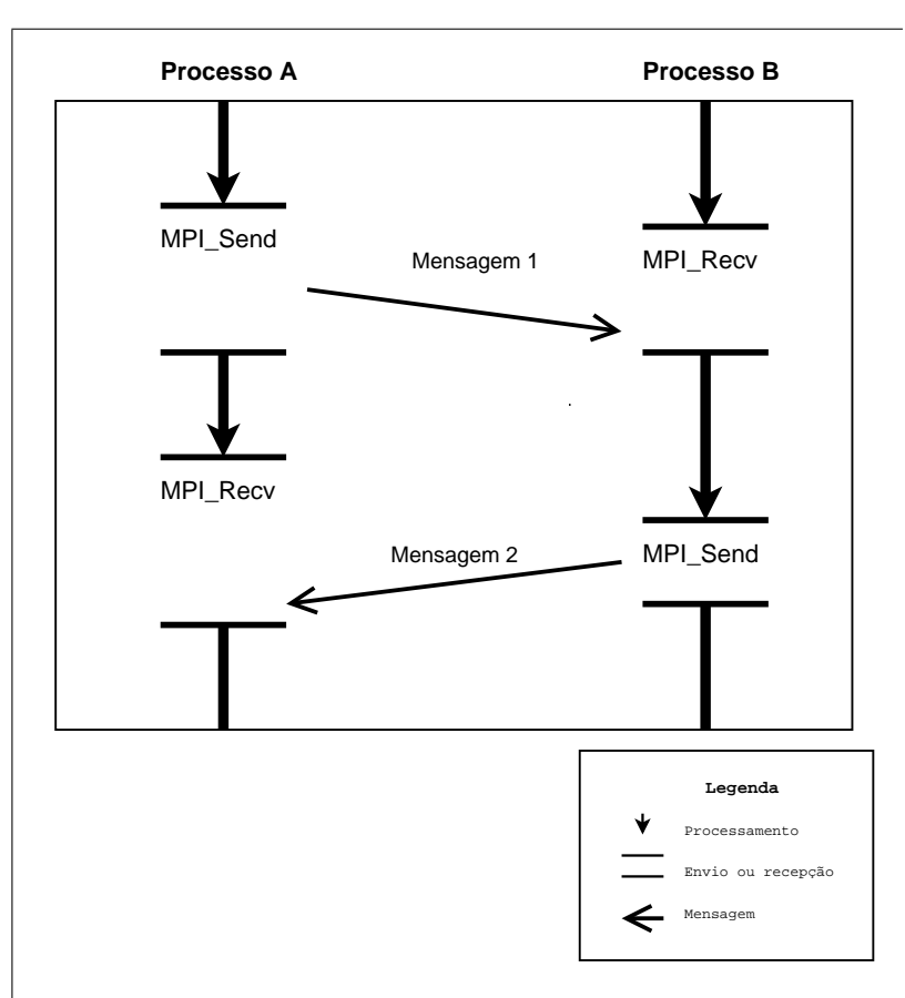
Figura 3.1 – Funcionamento do MPI_Send e do MPI_Recv
