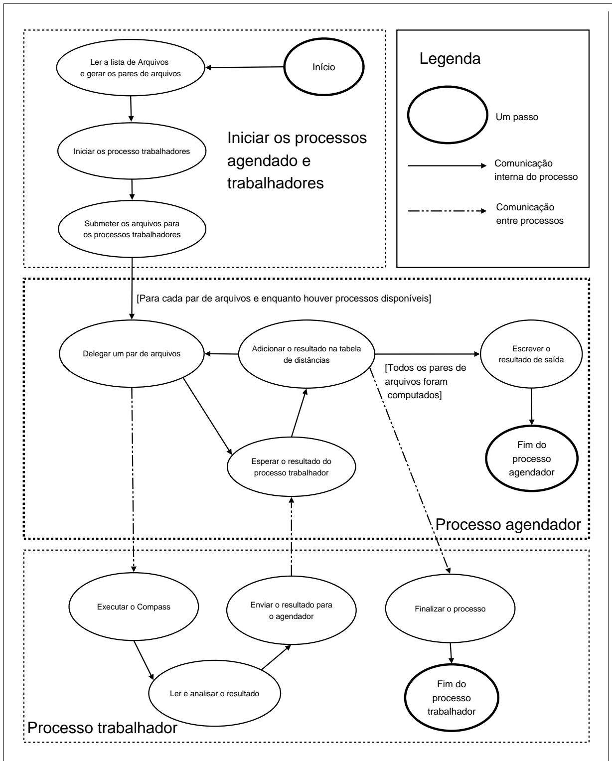
Figura 6.1 – Sequências de execução do agendador de múltiplas execuções do compass
