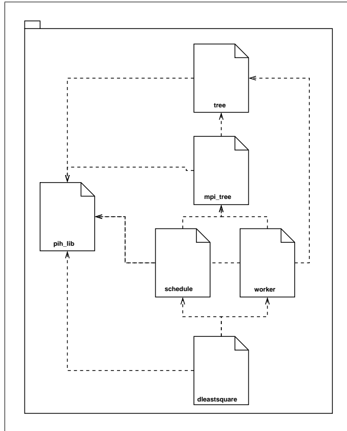
Figura 7.8 – Principais arquivos da implementação
