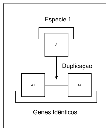
Figura 2.3 – Duplicação gênica
