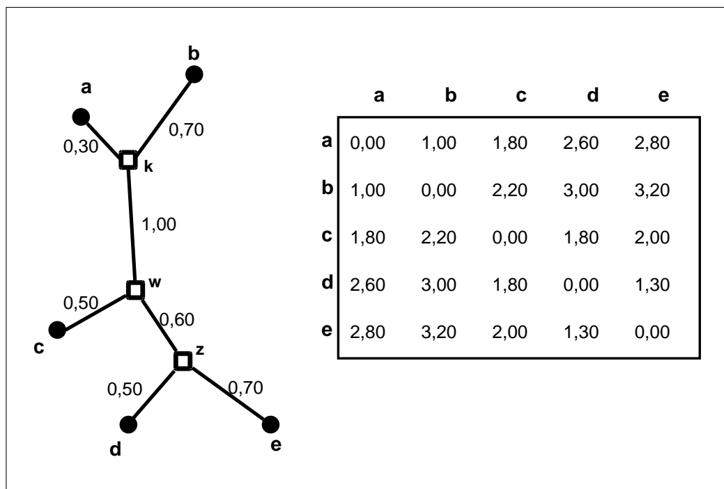
Figura 7.1 – Árvore ótima
