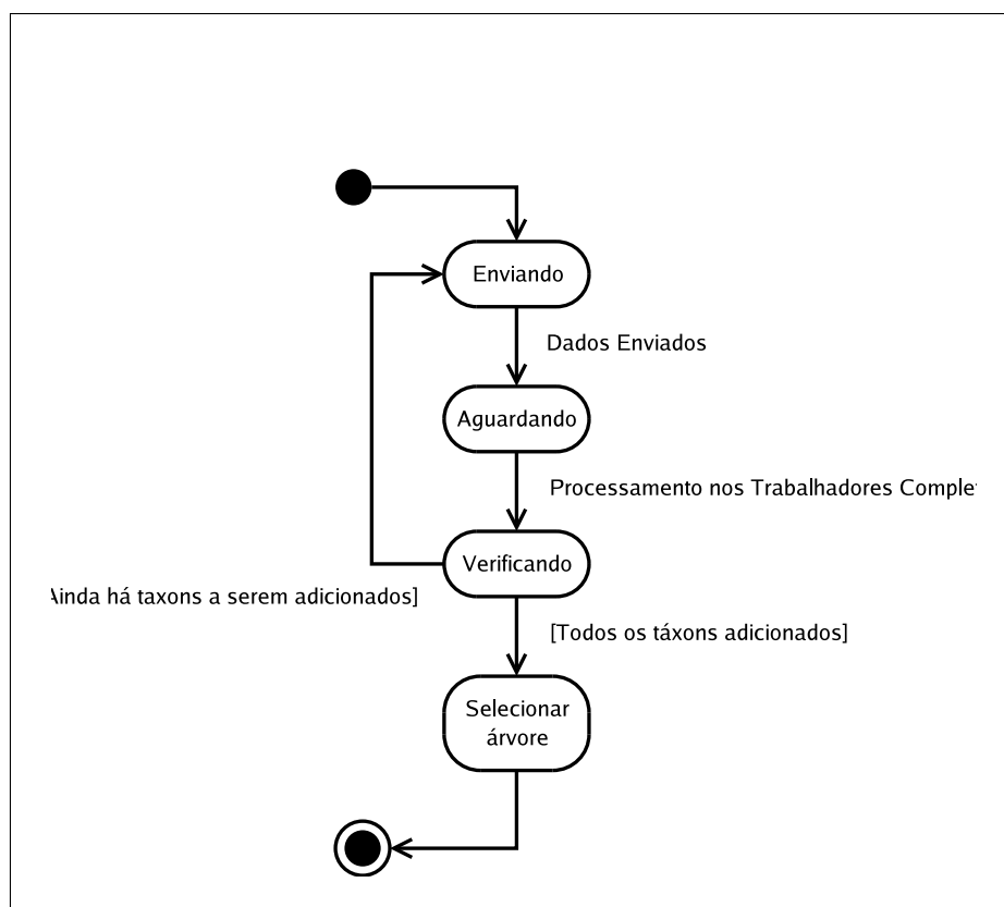
Figura 7.5 – Diagrama de estados do processo agendador
