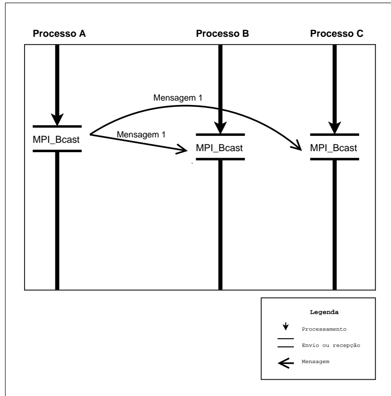
Figura 3.4 – Envio de dados a diversos nós utilizando broadcast
