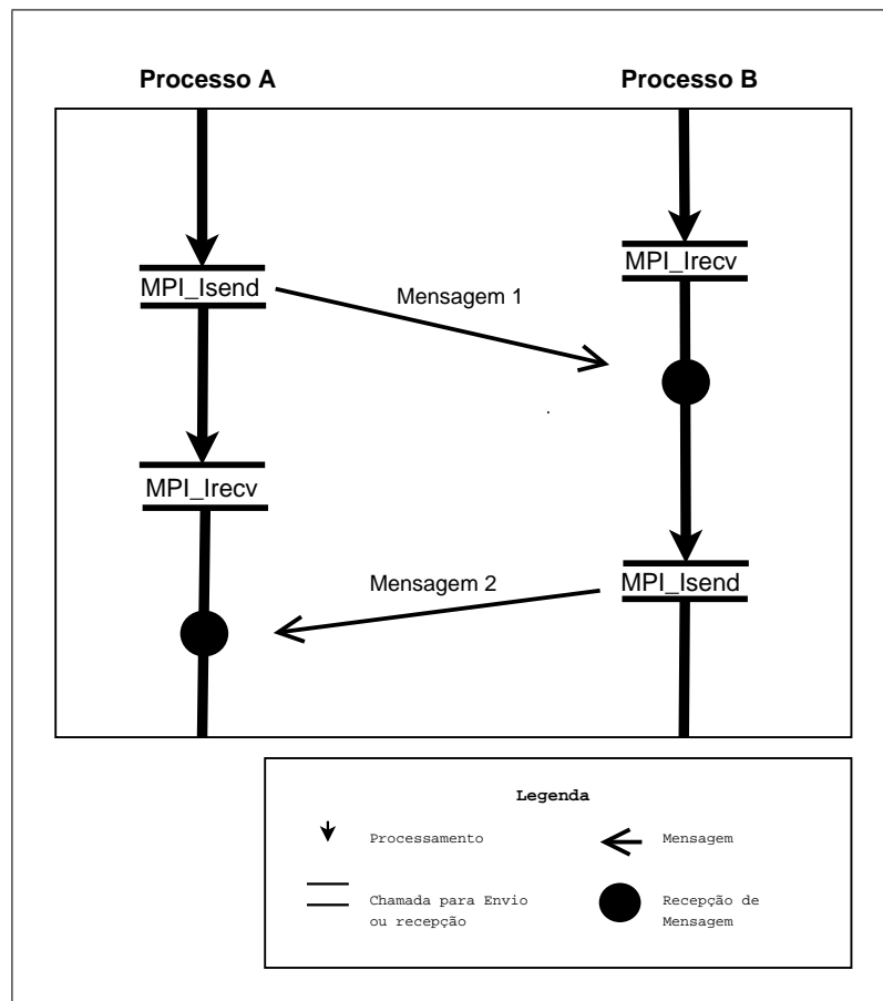
Figura 3.2 – Funcionamento do MPI_Isend e do MPI_Irecv
