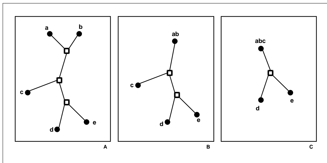
Figura 7.2 – Poda de uma árvore
