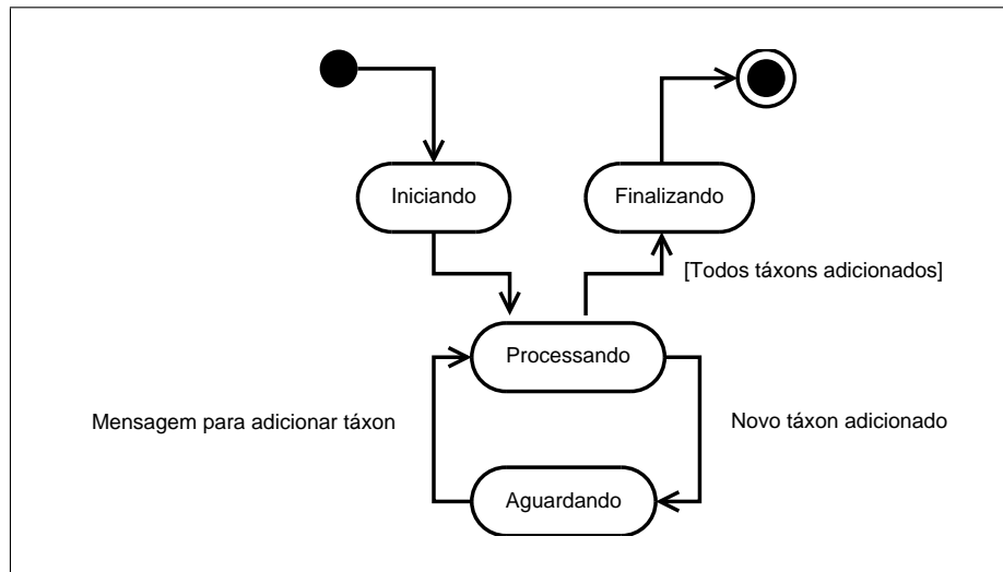
Figura 7.6 – Diagrama de estados dos processos agendadores
