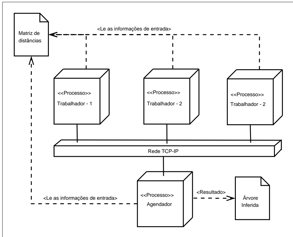
Figura 7.7 – Diagrama de distribuição do algoritmo
