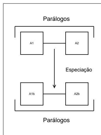
Figura 2.6 – Genes par logos
