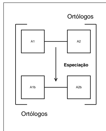
Figura 2.7 – Genes ortólogos
