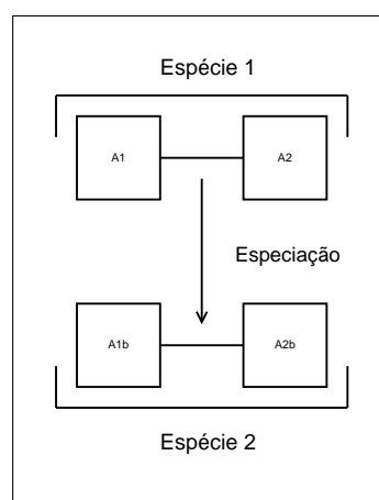
Figura 2.5 – Resultado da especia o nos genes
